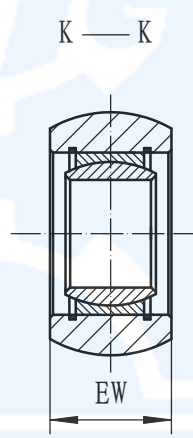
关节轴承式结构
