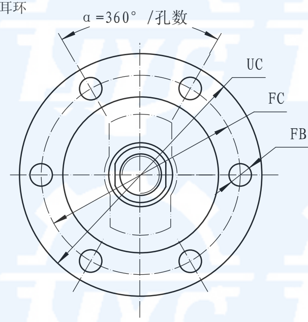
无油润滑衬套式结构
