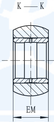
无油润滑衬套式结构
