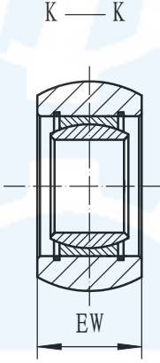
关节轴承式结构
