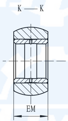
无油润滑衬套式结构
