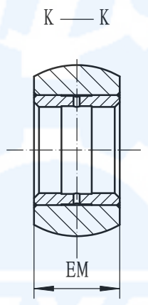
无油润滑衬套式结构
