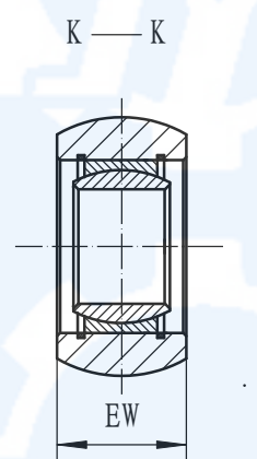
关节轴承式结构
