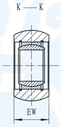
关节轴承式结构
